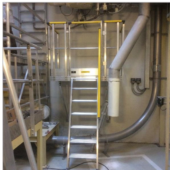
Plateforme avec échelle à marches pour accès poste de contrôle chaîne de production.
