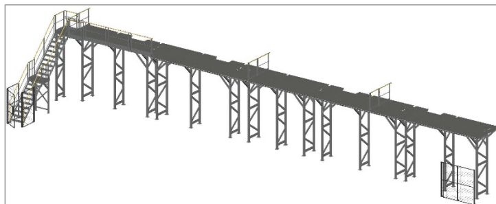
Vue 3D de l'ensemble de la passerelle
