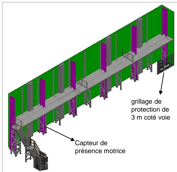
Présentation de l'implantation de l'ensemble escalier + passerelle dans la structure du bâtiment
