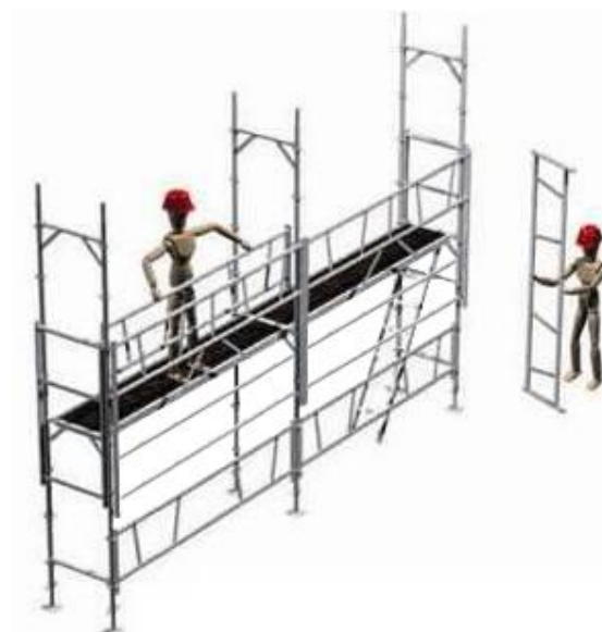
9 - Mise en place des garde-corps standard pour le niveau N
