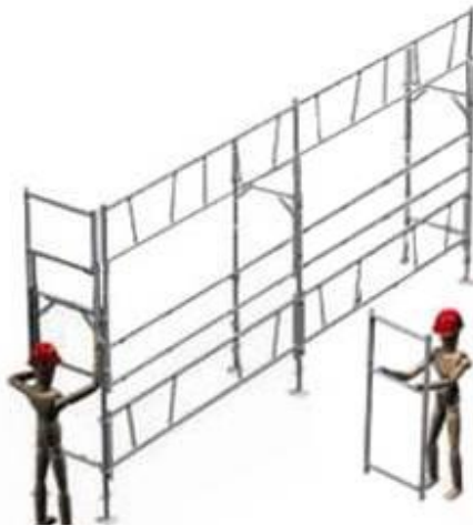
6 - Mise en place des garde-corps d'extrémité monobloc depuis le niveau 0 pour le niveau N+1
