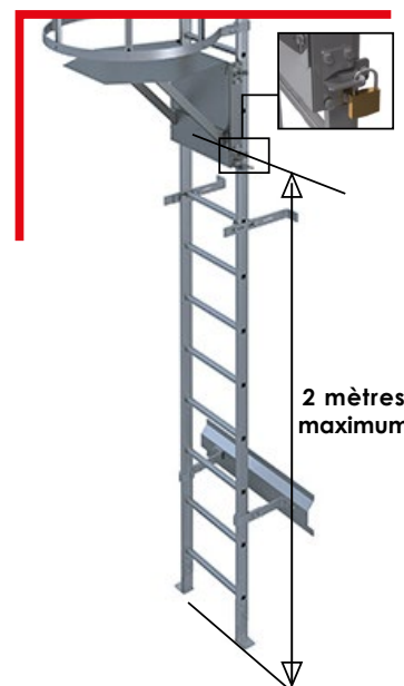
Porte de condamnation + opercule
