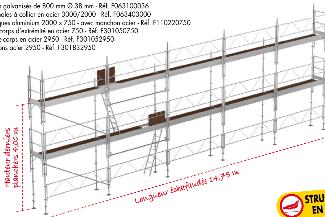
Garde-corps standard (voir p. 19)
