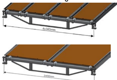
Plateforme largeur 1450
