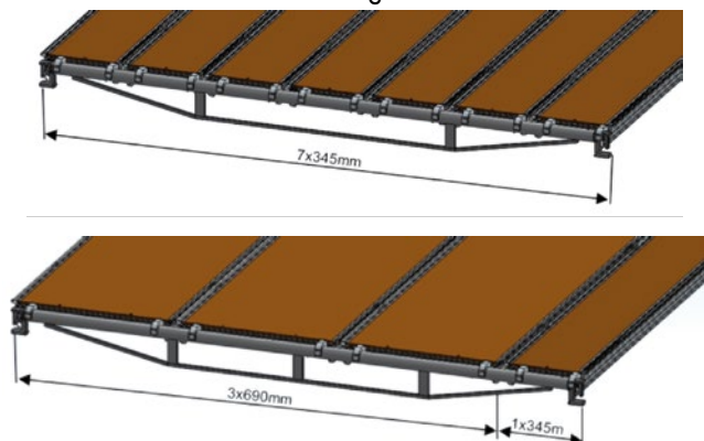
Plateforme largeur 2450
