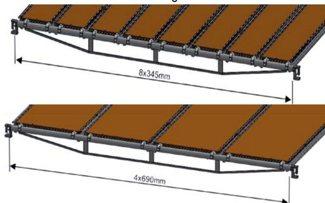
Plateforme largeur 2950
