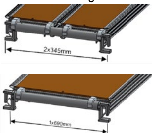
Plateforme largeur 750
