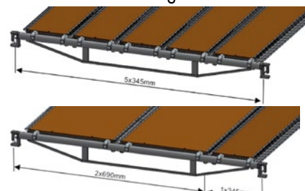
Plateforme largeur 1950
