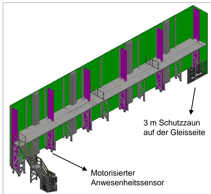
Darstellung des Aufbaus des Treppenhauses und der Bühne in der Gebäudestruktur
