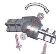
11 Beweglich Verbindung Zwischenleiste Ref. F191000015
